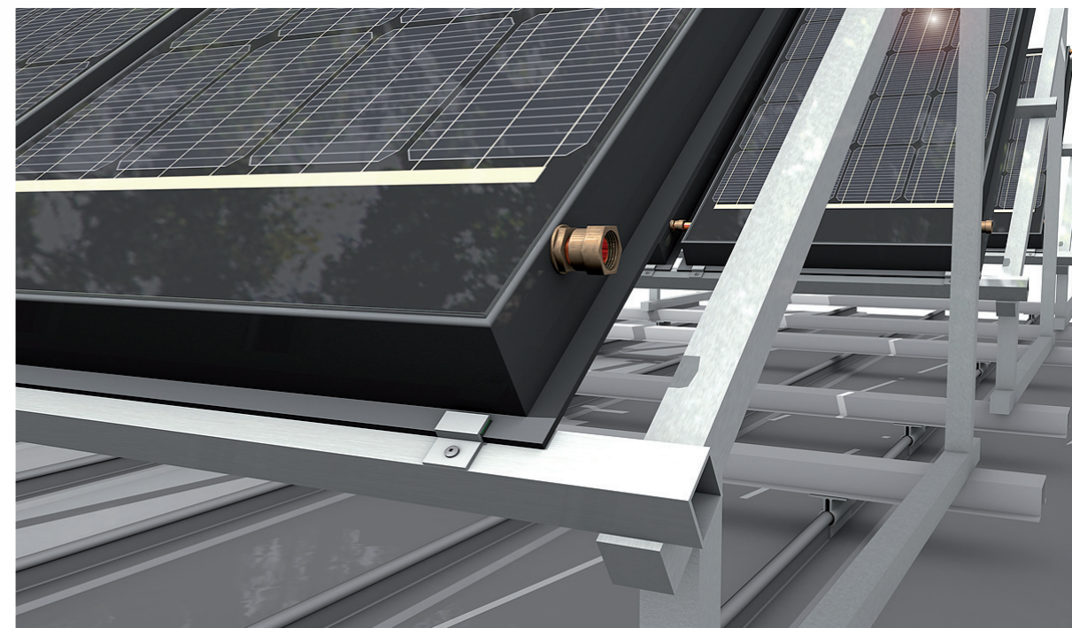
Montagedetail für stehende PIK ® Kombi-Solar-Kollektoren
